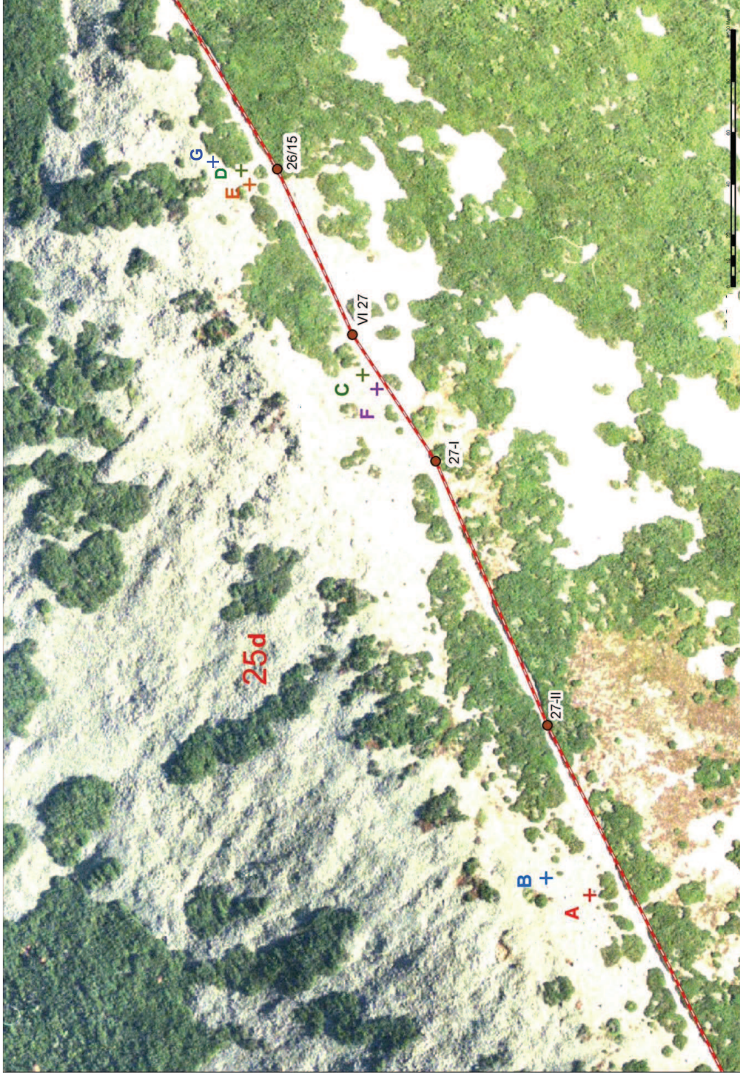
Ryc. 2. Lokalizacja badanych powierzchni na Czarnym Grzbiecie na tle ortofotomapy.
